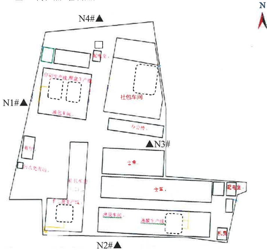
噪声检测点位示意图 检测（采样）时间（2024.09.03）
